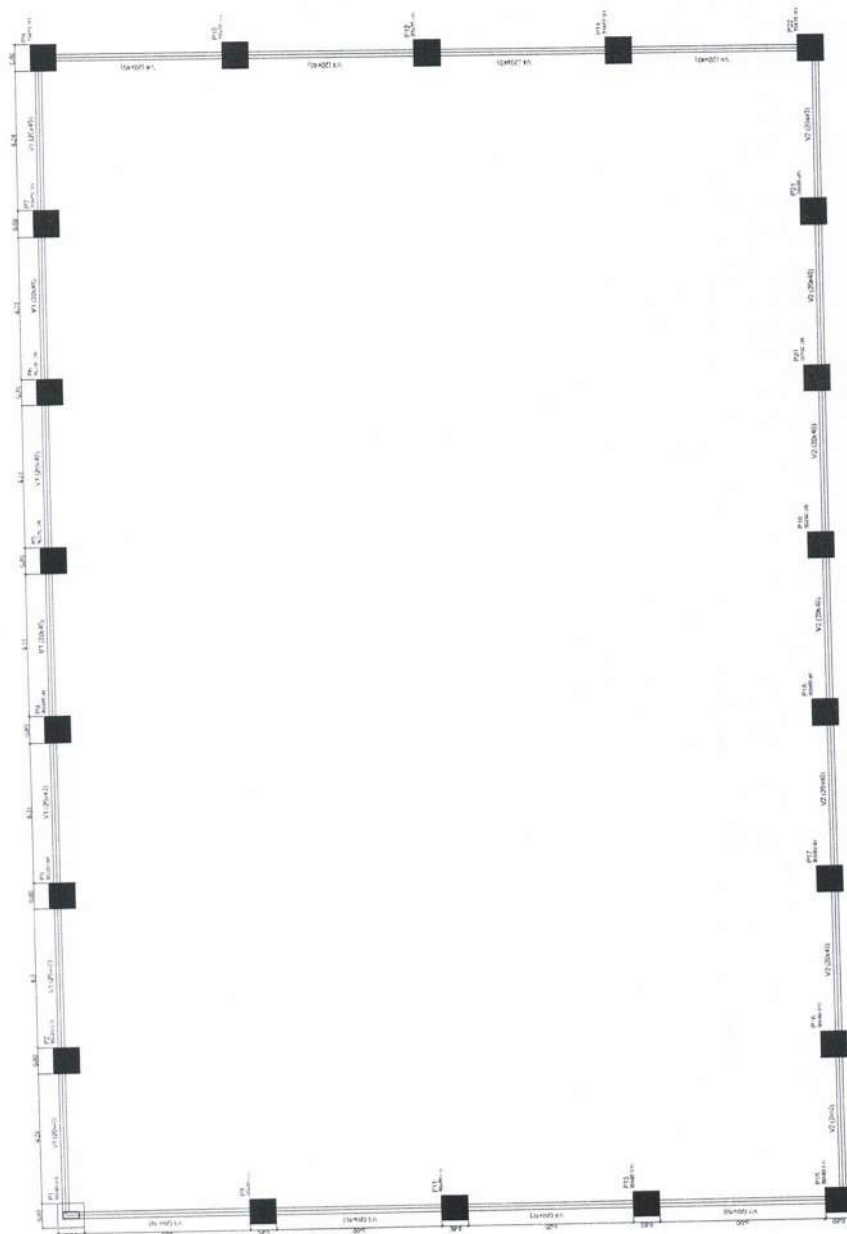
PLANTA DE FORMA DA VIGA BALDRAME ESCALA 1:75
