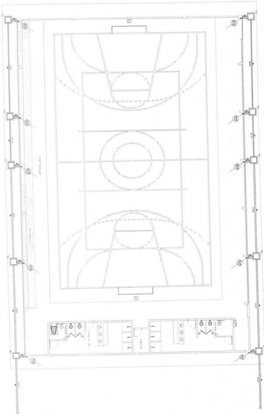
PLANTA BAIXA ESCALA 1/5
