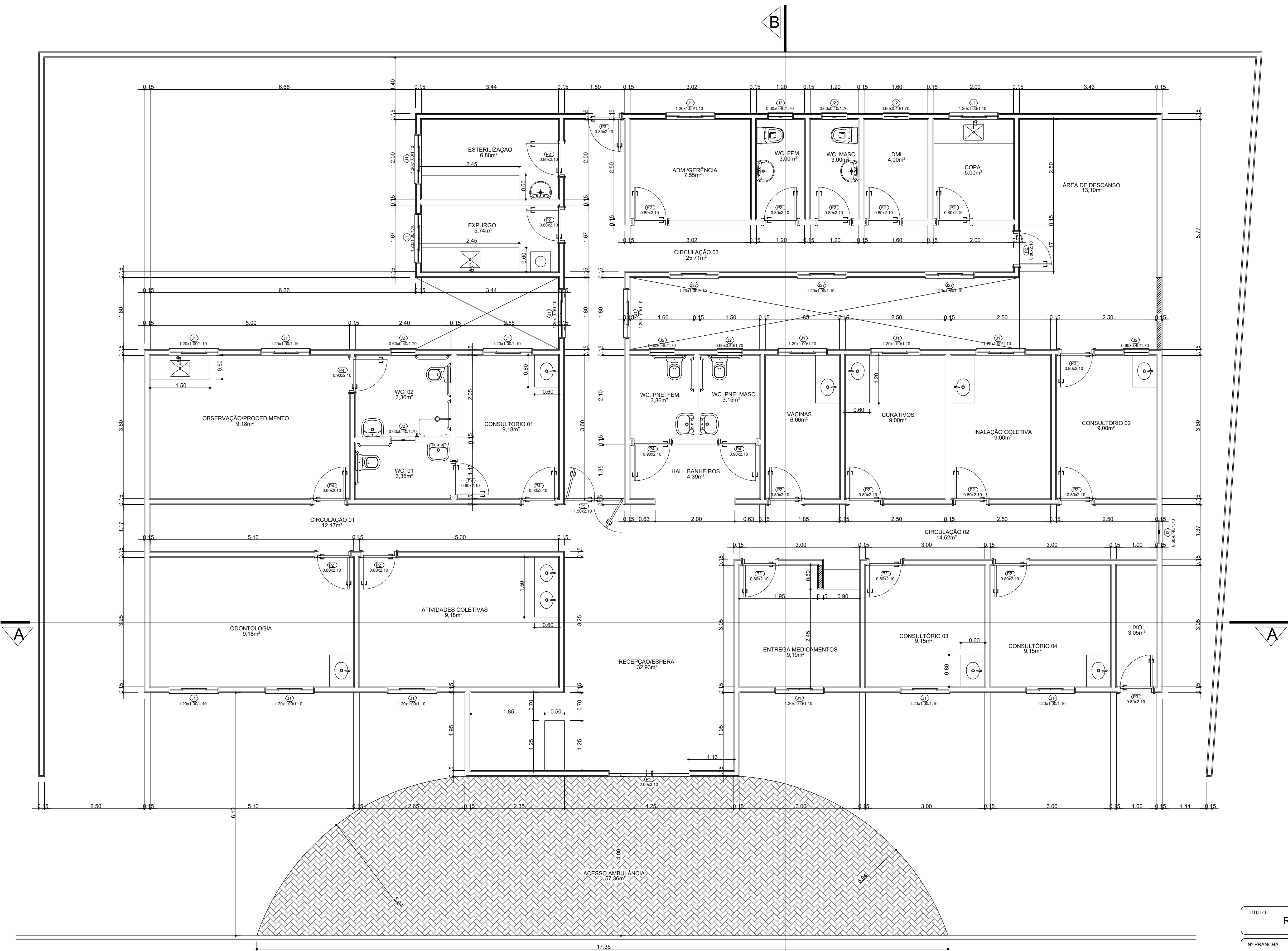
PLANTA BAIXA
